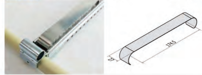
BS-A 滑輪煞車片 單件重量：28克 每箱數量：240pcs
