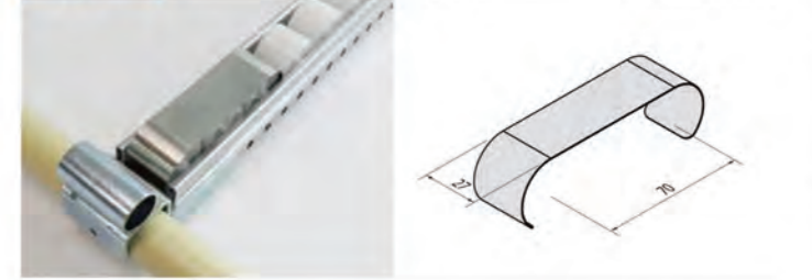
BS-A1 滑輪煞車片 單件重量：15克 每箱數量：240pcs
