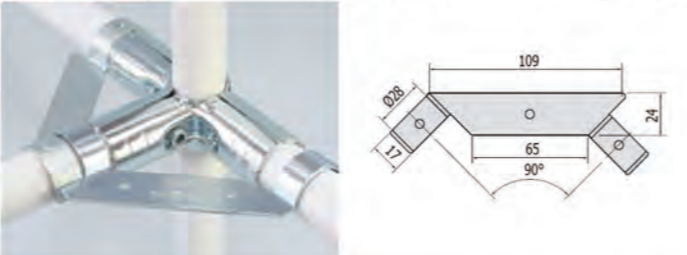
D-CSP 固定角落用金屬片 單件重量：69克 每箱數量：100pcs
