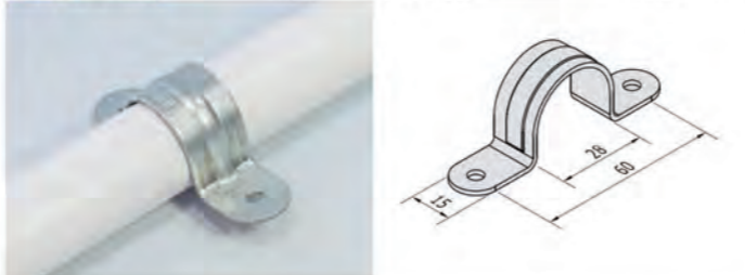
S.M-C 雙邊固定管夾 單件重量：17克 每箱數量：300pcs
