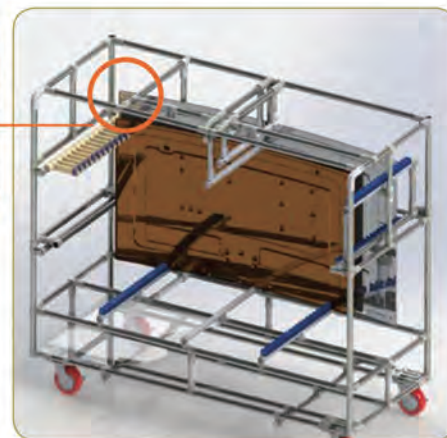
項目名稱：封底 零件：STS管，橡膠導軌 (G型)， DJP-400/400S 負載數量：20EA
