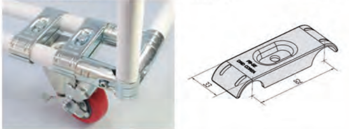
EF-1000A 腳輪金屬固定片 單件重量：102克 每箱數量：150pcs
