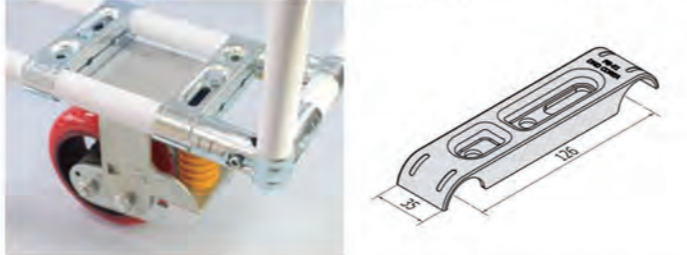
EF-1000B 腳輪金屬固定片 單件重量：136克 每箱數量：120pcs
