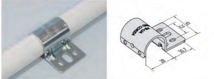
PB-UA 單邊固定管夾(寬版) 單件重量：63克 每箱數量：150pcs
