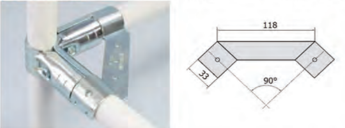
B.F.C.M-A 雙邊固定管夾 單件重量：97克 每箱數量：100pcs
