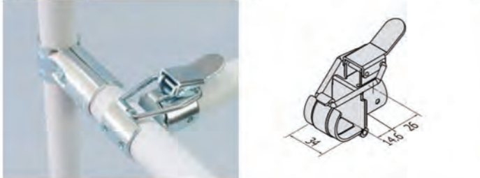
LM-01 易拆除鎖扣 單件重量：151克 每箱數量：50pcs
