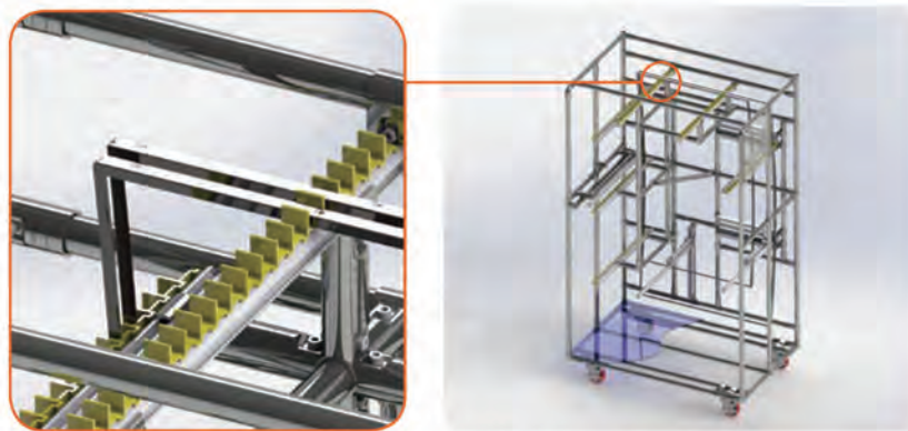
項目名稱：機箱頂部機箱 零件：STS管，AL2820， 橡膠導軌 (FSB-2) 負載數量：23EA
