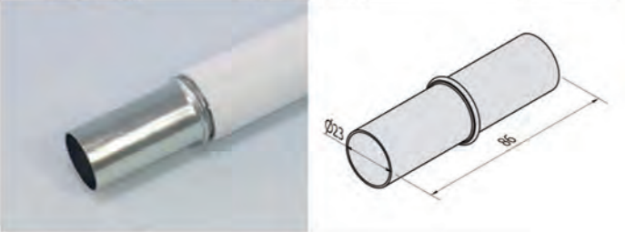
PB-CA 積木管接頭 單件重量：72克 每箱數量：100pcs
