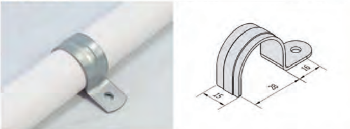
S.M-B 單邊固定管夾 單件重量：27克 每箱數量：200pcs
